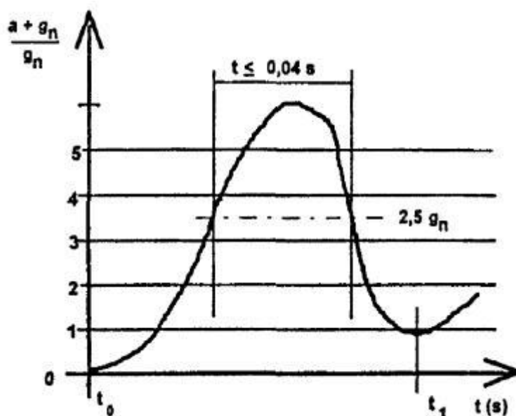
Рис. 1. График торможения
